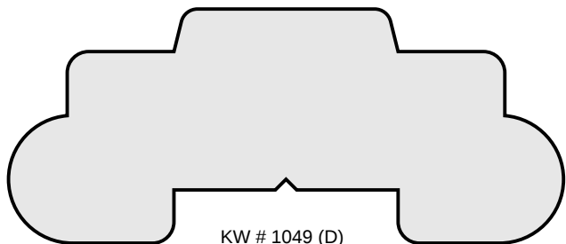
KW # 1049 (D) 1-3/8" x 3-1/4"
